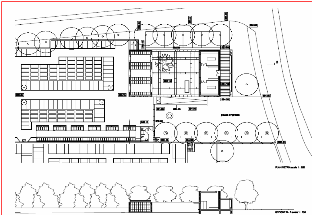
La zona inferiore, angolo tra Via Povrò e Via Martignoni, planimetria
