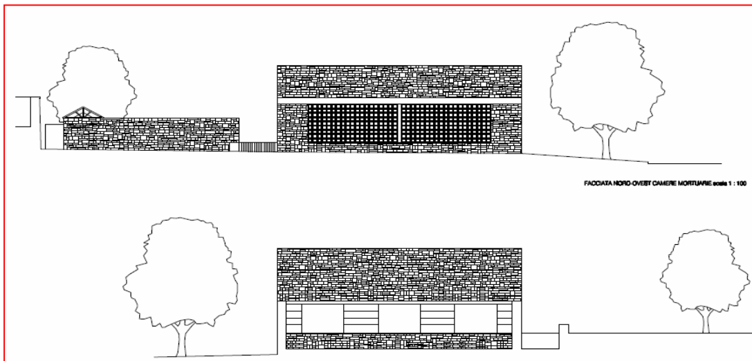
Viste prospettiche camere mortuarie
