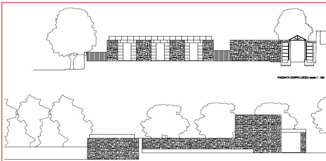
Prospetto corpo loculi (frontale interno al cimitero e laterale su asse pedonale interno)
